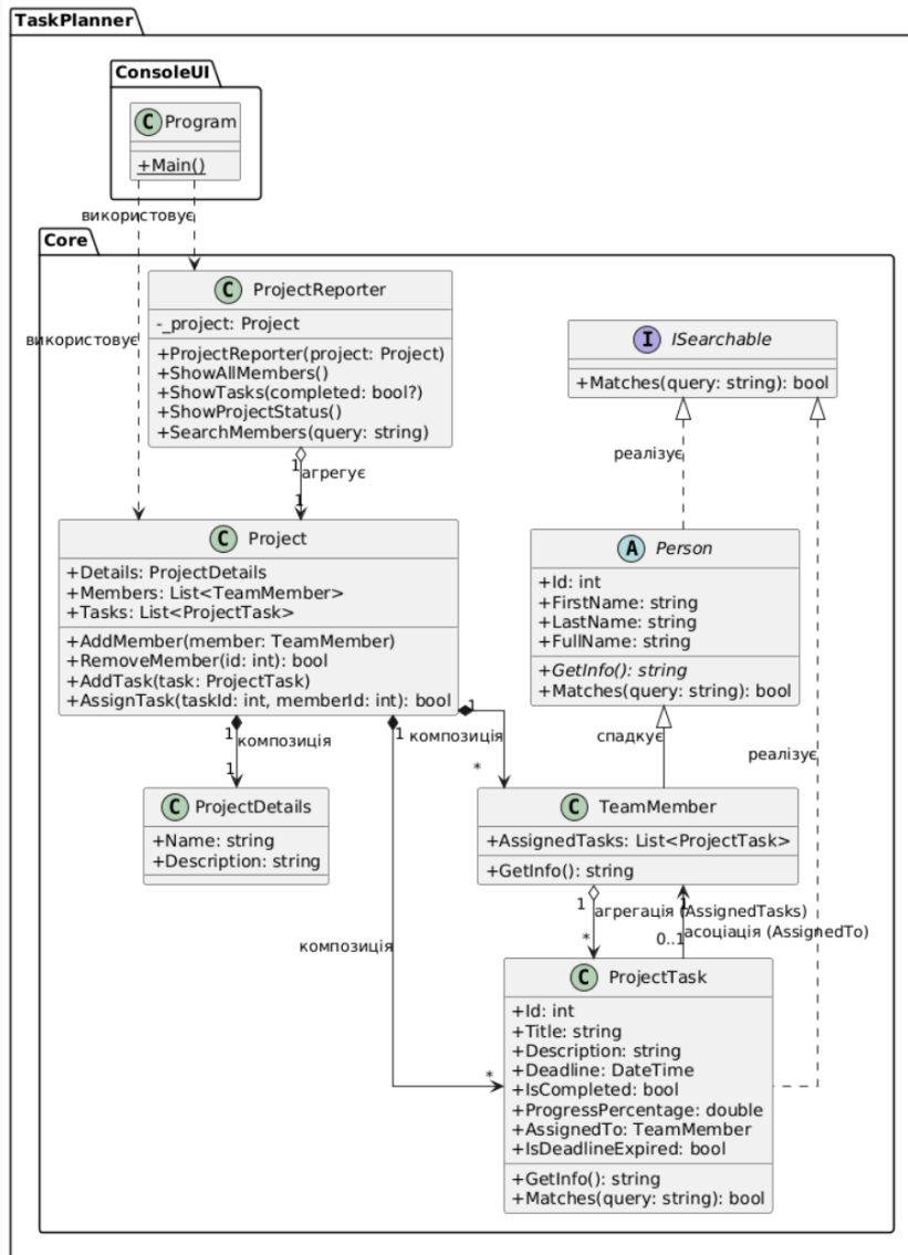
Діаграма класів: Планувальник завдань (Багатошарова архітектура)
